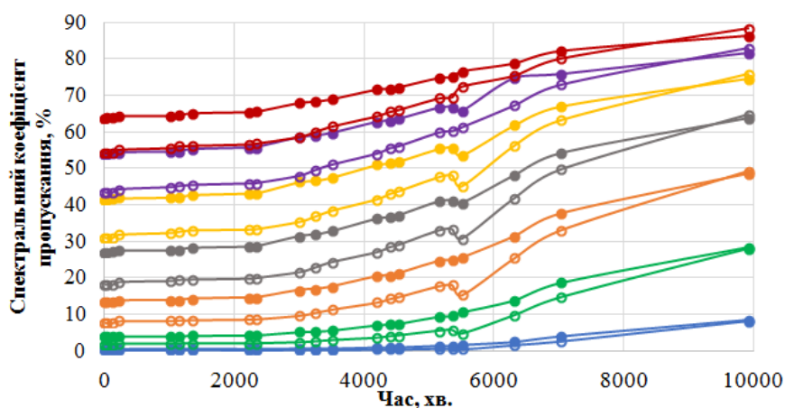
Рис. 6. Залежність спектральних коефіцієнтів пропускання для НФ ізопропанол/ \text{Al}_2\text{O}_3 0.5 мас. %, що були приготовані за технологією 2:
