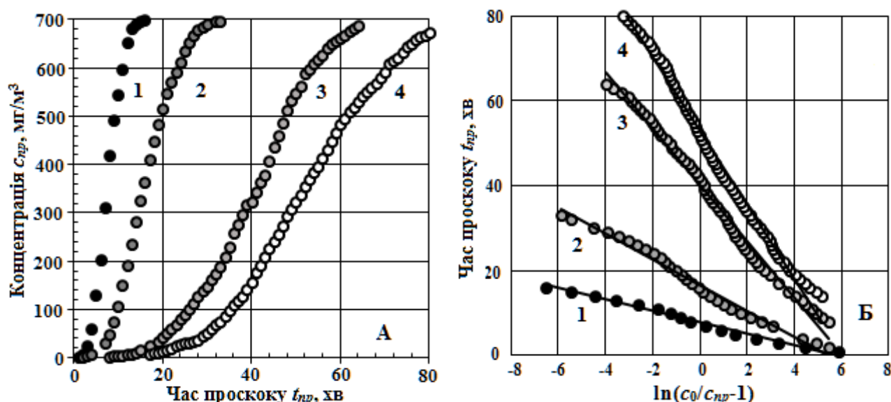
Рис. 2. Криві проскоку аміаку через шар ІВХС для різних значень відносної вологості ГПС: А – залежність c_{np}(t_{np}) , Б – залежність t_{np} [\ln(c_0/c_{np} - 1)] .
