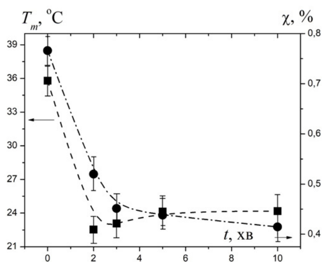
Рис. 5. Залежність температури плавлення та ступеня кристалічності від часу змішування для полімерних нанокомпозитів на основі ПЕГ та ОММТ.
