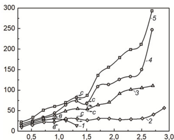
Рис.7. Розповсюдження полум'я в аерозависах частинок ПАМ-4 ( d = 14.5 \text{ мкм} ) в трубах. L = 3.5 \text{ м} , d = 5.6 \text{ см} ; B : 1 - 140 \text{ г/м}^3 ; 2 - 160 \text{ г/м}^3 ; 3 - 150 \text{ г/м}^3 ; 4 - 300 \text{ г/м}^3 ; 5 - 580 \text{ г/м}^3 .
