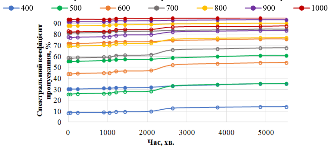
Рис. 7. Залежність спектральних коефіцієнтів пропускання для НФ ізопропанол/ \text{Al}_2\text{O}_3 0,2 мас. %, що були приготовані за технологією 3:
