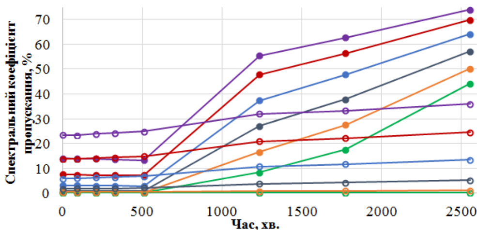
Рис. 5. Залежність спектральних коефіцієнтів пропускання для НФ ізопропанол/ \text{Al}_2\text{O}_3 0,5 мас. %, що були приготовані за технологією 2:
