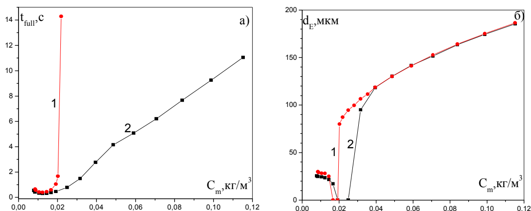
Рис.4. Залежність часу повного перетворення і критичного діаметра d_E від масової концентрації палива в газозависі при T_{g\infty}=1250 К. 1 – без урахування зовнішнього тепломасообміну; 2 – з урахуванням.
