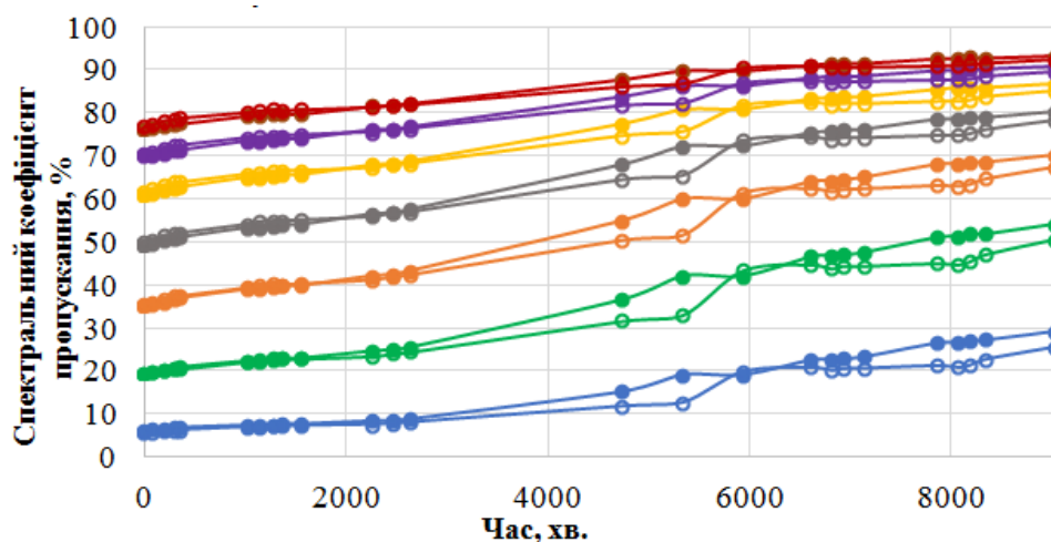
Рис. 4. Залежність спектральних коефіцієнтів пропускання для НФ ізопропанол/ \text{Al}_2\text{O}_3 0,2 мас. %, що були приготовані за технологією 1:
