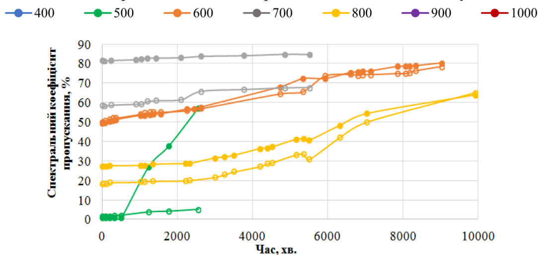
Рис. 8. Залежність спектральних коефіцієнтів пропускання світла з довжиною хвилі 700 нм для НФ ізопропанол/ \text{Al}_2\text{O}_3 , що були приготовані за різними технологіями: ● – недеаеровані НЧ, ○ – деаеровані НЧ;
