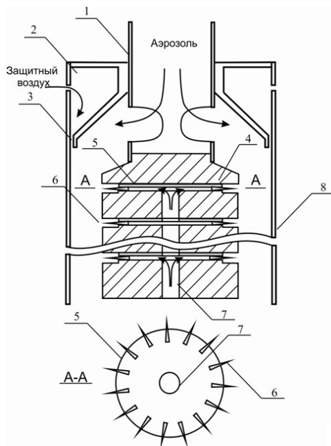
Рис.1 Схема конструкции ионизатора [7].
